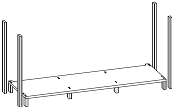
Fußgestell Für 3 Unterschrankelemente 1 Bodenplatte mit höhenverstellbaren Füßen inkl. Stollen inkl. Fußkantenschutz
