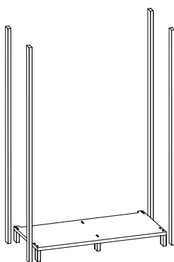
Fußgestell für 2 Hochschränkelemente 1 Bodenplatte mit höhenverstellbaren Füßen inkl. Stollen inkl. Fußkantenschutz
