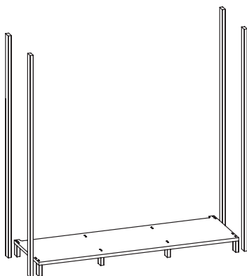
Fußgestell für 3 Hochschränkelemente 1 Bodenplatte mit höhenverstellbaren Füßen inkl. Stollen inkl. Fußkantenschutz
